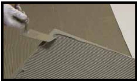
Fig.29 - Applicare l’adesivo con la tecnica della doppia spalmatura e cioè stendendo l’adesivo a letto pieno sul supporto, usando una spatola a denti distanziati tra loro di almeno 6 mm (ad esempio Raimondi art.138HFV6). Quindi applicare l’adesivo anche sul retro della lastra, utilizzando una spatola con denti da 3 mm. Ricordarsi di ripassare l’adesivo sul perimetro della lastra.
